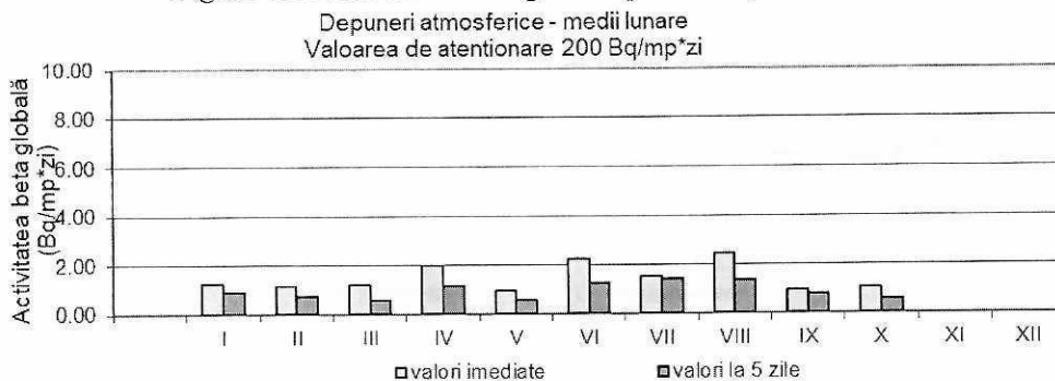
Figura 15. Activitatea beta globală pentru depuneri atmosferice
