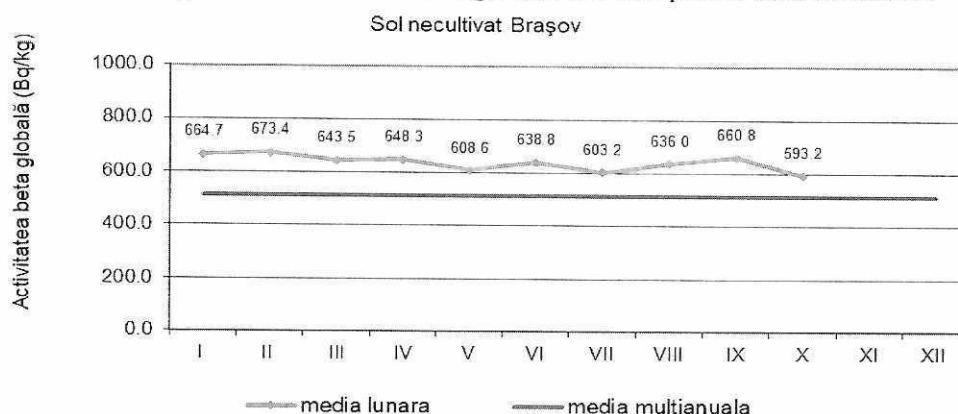
Figura 19. Activitatea beta globală la 5 zile pentru solul necultivat
