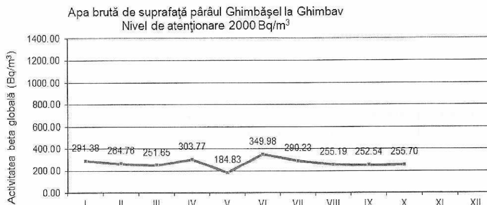
Figura 16. Activitatea beta globală imediată pentru apa de suprafață Pârâul Ghimbășel
