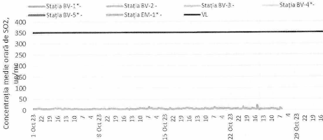
Figura 1. Evoluția mediilor orare de SO 2 în luna octombrie
