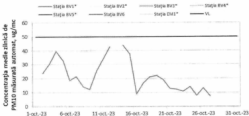
Figura 8. Evoluția mediilor zilnice de PM 10, metoda automată, în luna octombrie
