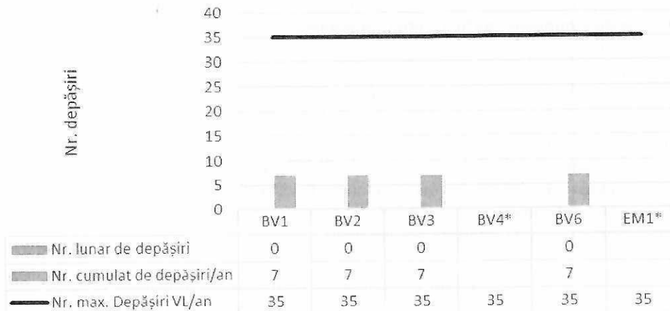
Figura 7. Numărul lunar și cumulat de depășiri ale valorii limită zilnice la PM10
