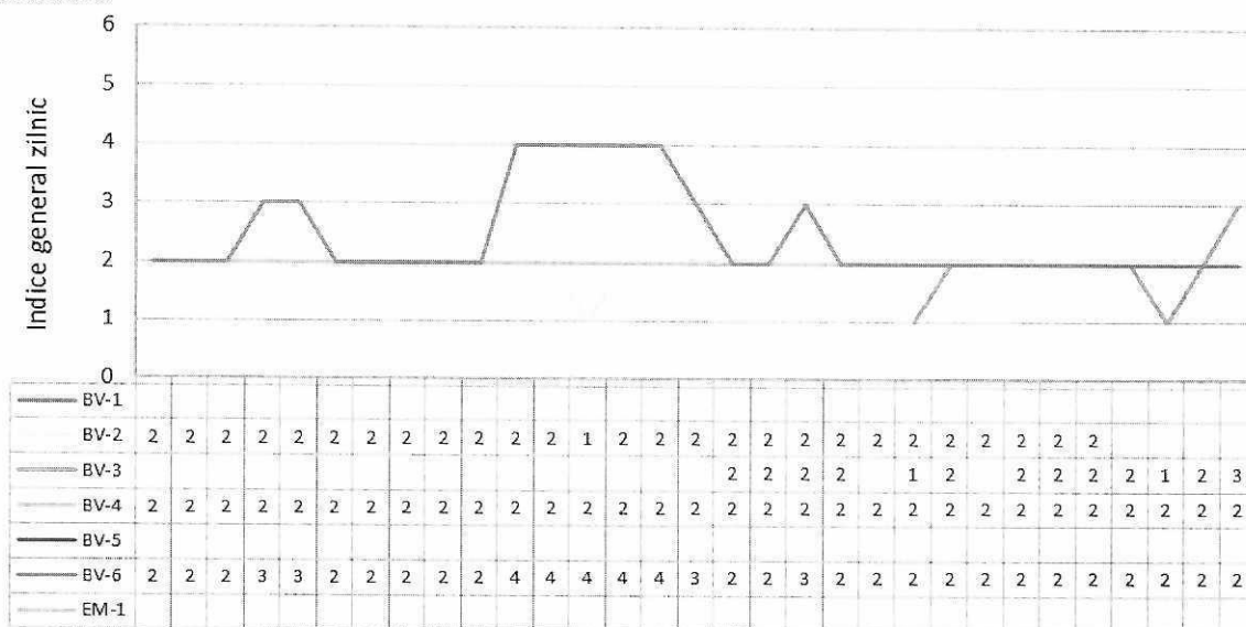
Figura 11. Evoluția indicelui general de calitatea aerului din rețeaua locală de monitorizare a calității aerului
