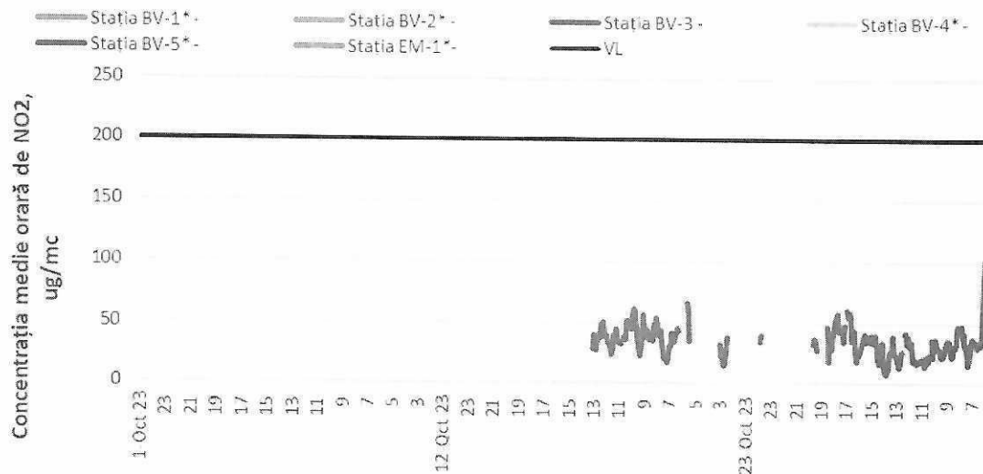
Figura 3. Concentrații medii orare de \text{NO}_2 în luna octombrie 2023
