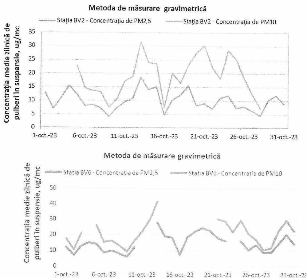
Figura 9. Evoluția mediilor zilnice de PM 2,5 și PM10 în luna octombrie
