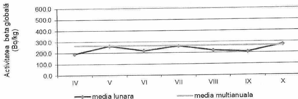
Figura 20. Activitatea beta globală la 5 zile pentru vegetația spontană Vegetație spontană Brașov
