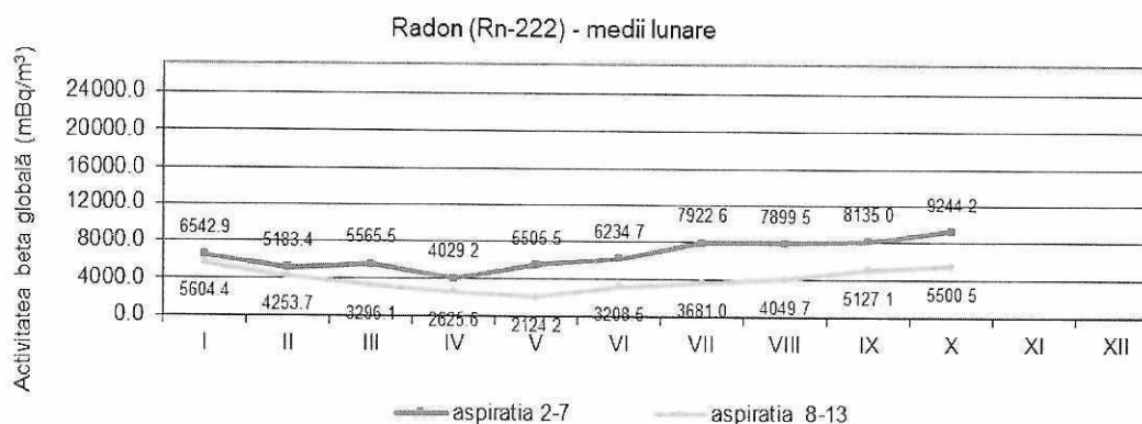
Figura 13. Activitatea calculată a Radonului
