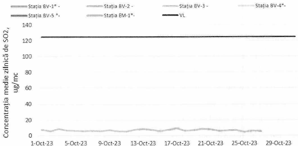
Figura 2. Evoluția mediilor zilnice de SO 2 în luna octombrie
