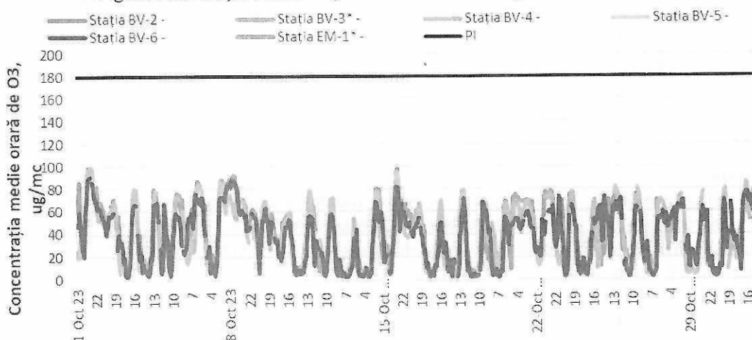
Figura 5. Evoluția concentrațiilor medii orare de O 3 în luna octombrie
