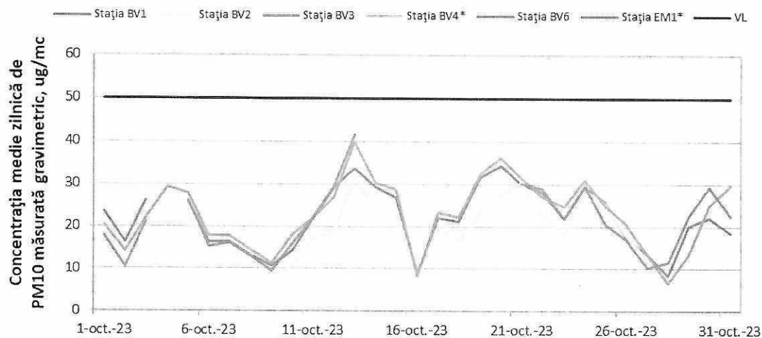
Figura 6. Evoluția mediilor zilnice de \text{PM}_{10} (gravimetric) în luna octombrie
