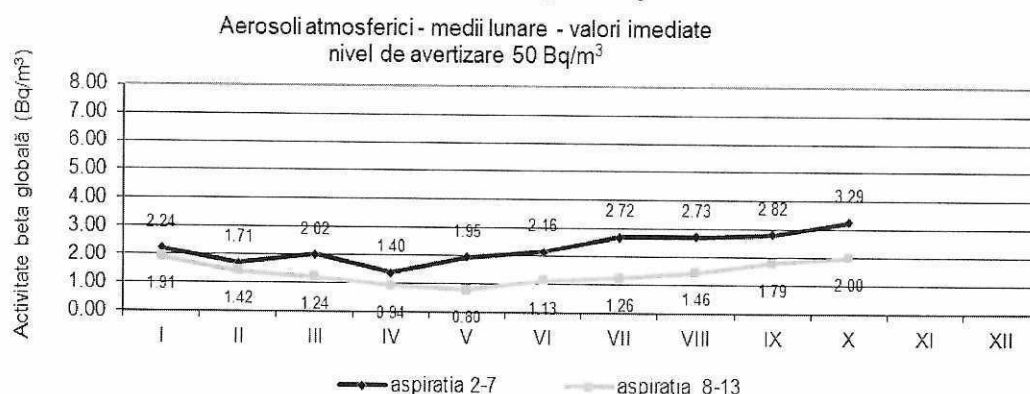
Figura 12. Activitatea beta globală pentru aerosoli atmosferici
