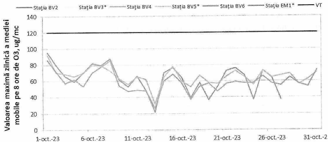
Figura 4. Evoluția concentrațiilor maximelor zilnice ale mediilor mobile pe 8 ore de O 3 în luna octombrie
