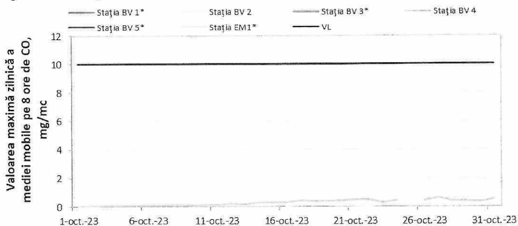
Figura 10. Evoluția maximelor zilnice ale mediei mobile de CO în luna octombrie
