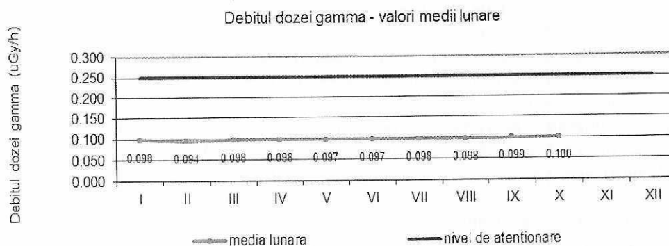
Figura 14. Debitul dozei gamma
