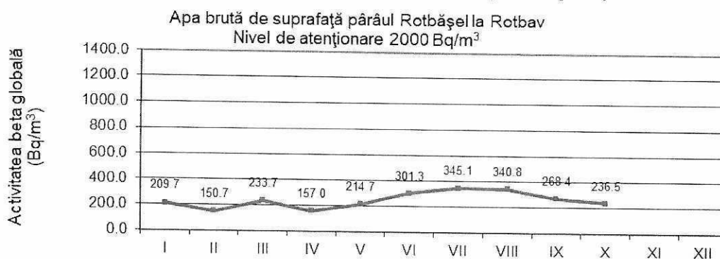
Figura 17. Activitatea beta globală la 5 zile pentru apa de suprafață-Pârâul Rotbășel
