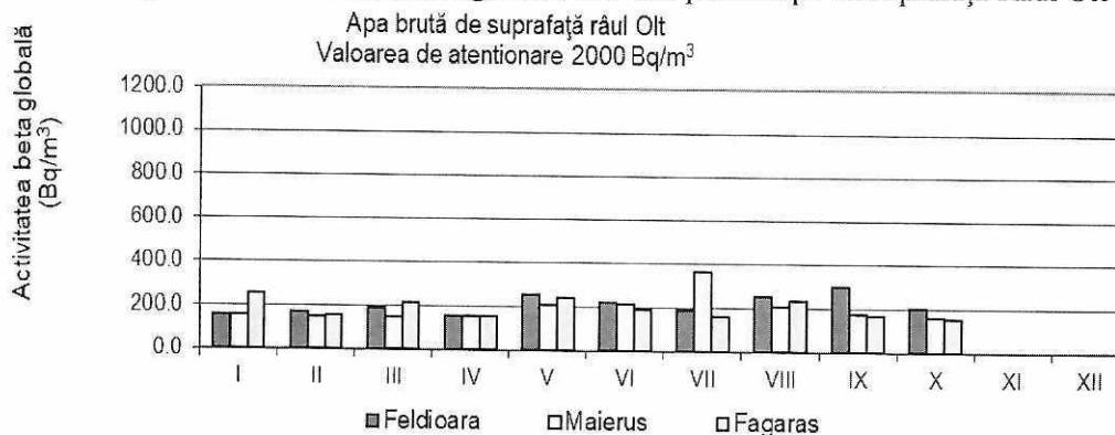
Figura 18. Activitatea beta globală la 5 zile pentru apa de suprafață Râul Olt
